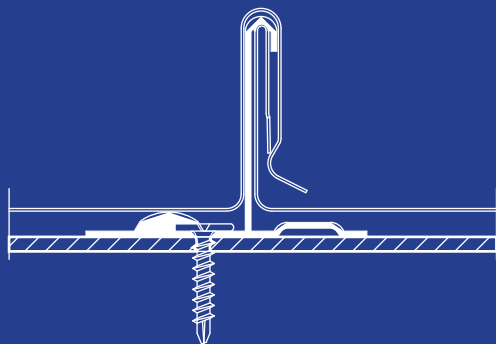
SnapLok Seam
